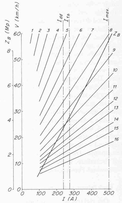
Bild 13. Bremskennlinien
