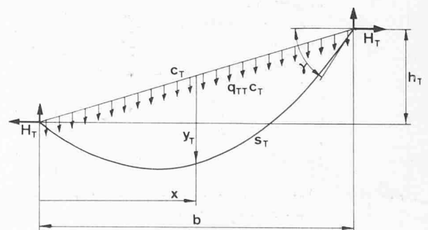
Bild 3. Tragseilkurve im Leerfeld
