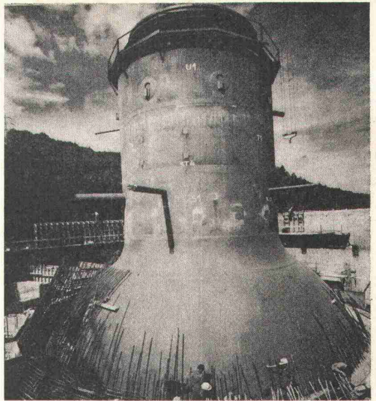
Wichtige Teile des Kernkraftwerkes Mühleberg wurden mit Sécheron-Elektroden geschweisst.
