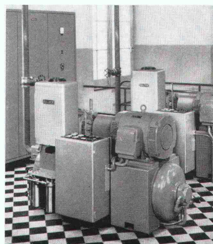
Rotations-Vielzellenverdichter
