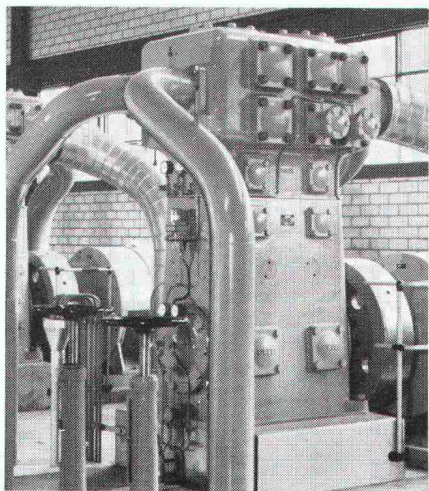
Labyrinthkolben-Kompressor
