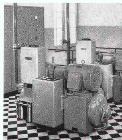
Rotations-Vielzellenverdichter
