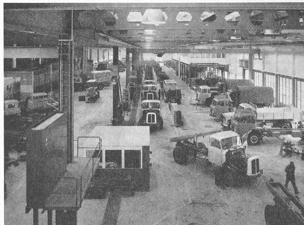
Bild 7. Blick in die neue Montagehalle, gesehen von Ost nach West. Links die Verlagsmontage, rechts die Chassismontage, im Vordergrund rechts die Nacharbeitsplätze, im Hintergrund das Montageband
