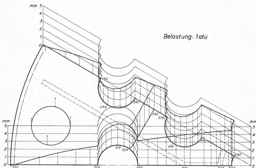
Bild 9. Tragplatte. Achsiale Verformung
