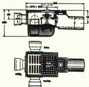
Kellerablauf «Junior» mit Rückstaudoppelschloss
