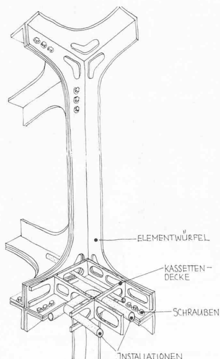
Biege feste Stahlwürfel-Rahmen als flexible Elemente im Zusammenbau und in der Nutzung (vorfabriziert, stapelbar)
