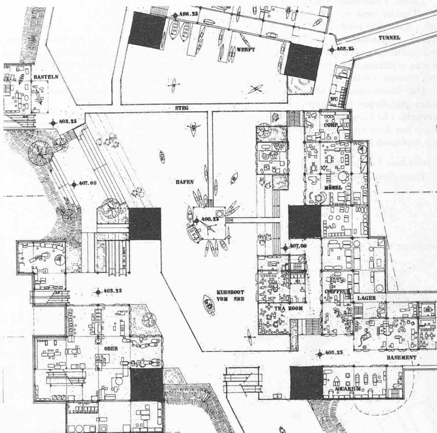
Teilplanung am Schanzengraben, Grundriss Basement
