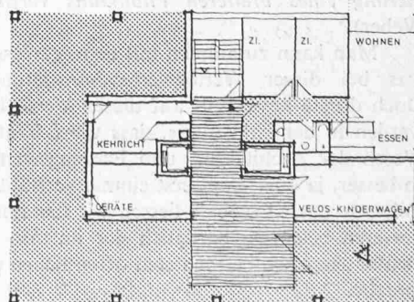
Erdgeschoss mit Wohnung zu 3\frac{1}{2} Zimmern und geräumiger Eingangshalle
