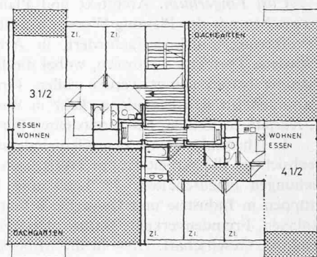
Dachgeschoss mit zwei Wohnungen zu 3\frac{1}{2} und 4\frac{1}{2} Zimmern
