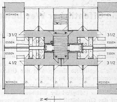
Erdgeschoss mit Wohnung zu 3\frac{1}{2} Zimmern und geräumiger Eingangshalle
