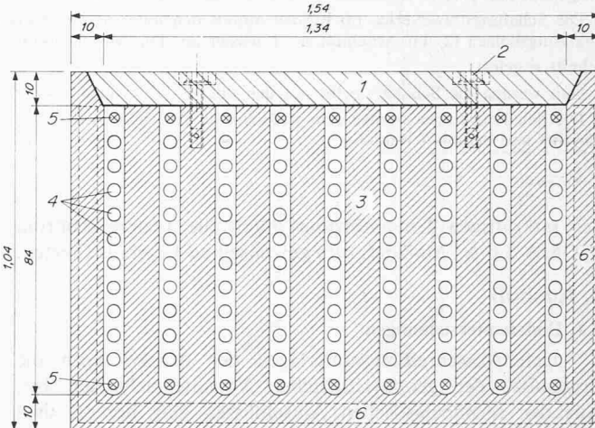
Bild 7. Querschnitt der ausgeführten Zugbänder. 1 Deckel, 2 Bolzen zum Festhalten der Deckel auf den Elementen, 3 kammförmiges Zugbandelement, 4 9×10 Trageile 1 1/8", 5 2×9 Spannglieder für die Eigenvorspannung, 6 nut- und kammförmig ausgebildete Stirnflächen. Die verbleibenden Hohlräume wurden mit Zementmörtel ausinjiziert
