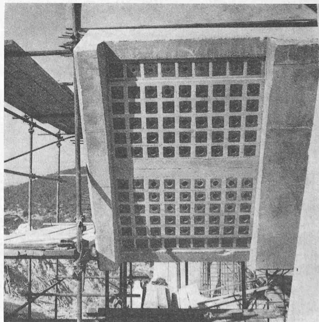
Bild 8. Verankerungsanordnung der 9×10 Trageile sowie der 2×9 Spannglieder für die Eigenvorspannung der Zugbandumhüllung im auskragenden Seilquerträgerteil
