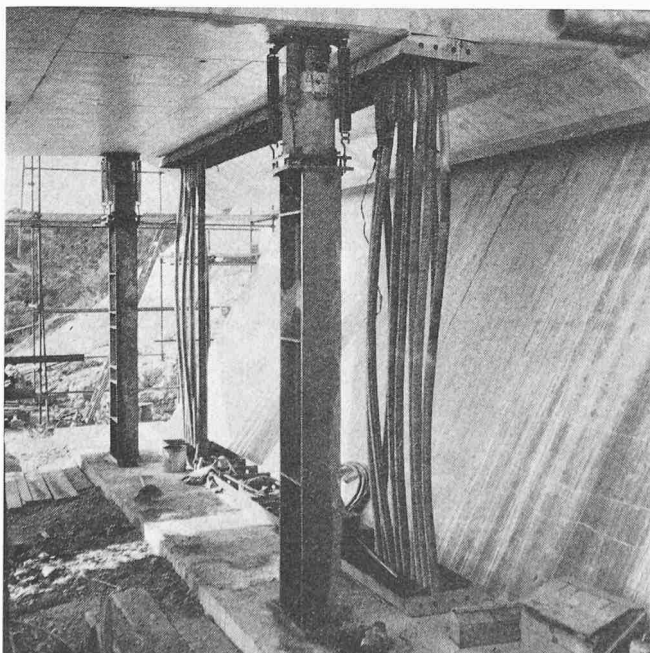
Bild 24. Auf der Auflagebank des Widerlagers A stehende Spriesse, welche das Gewicht des darüberliegenden Seilquerträgers abfangen. Am Kopf der Spriesse die 300-t-Stellingpressen, dank welchen die Lasten dauernd überwacht werden. Parallel zu den Spriessen die zum Teil noch ungespannten Vertikalkabel
