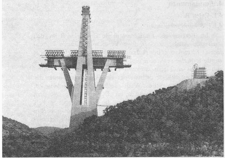
Bild 14. Die beiden Enden des Lehrgerüsts sind losgelöst und zu Vorbauwagen umgebaut. Rechts ist das im Bau begriffene Widerlager D ersichtlich mit den beiden Schleifen der späteren Vertikalkabel
