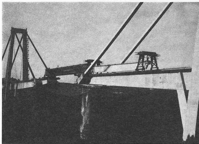
Bild 29. Der vordere Portalkran, an welchem einer der bergseitigen Träger aufgehängt ist, hat den Hilfsträger erreicht. Ein Teil des Grobsandes wird in das Wadibett auslaufen gelassen. Zwischen den beiden wadiseitigen Seilquerträgern ist das Auffangnetz gespannt. Die Zugbandelemente beim Pylon im Hintergrund sind noch nicht montiert
