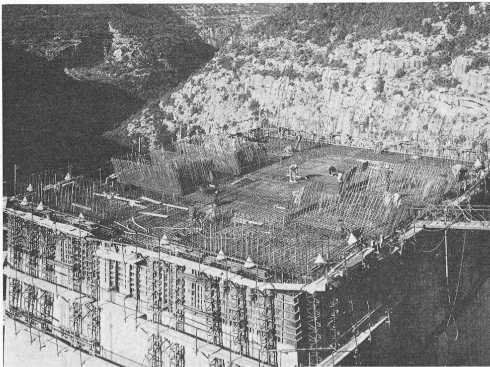
Bild 10. Armierung der Pylonsockeldecke. Die Anschlussstähle der Schräg- und Turmstützen ragen im Moment über die Arbeitsplattform hinaus.
