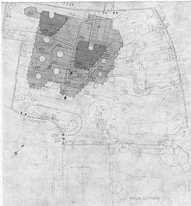
Lageplan 1:2500
