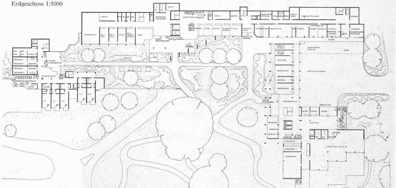
Erdgeschoss 1:1000
