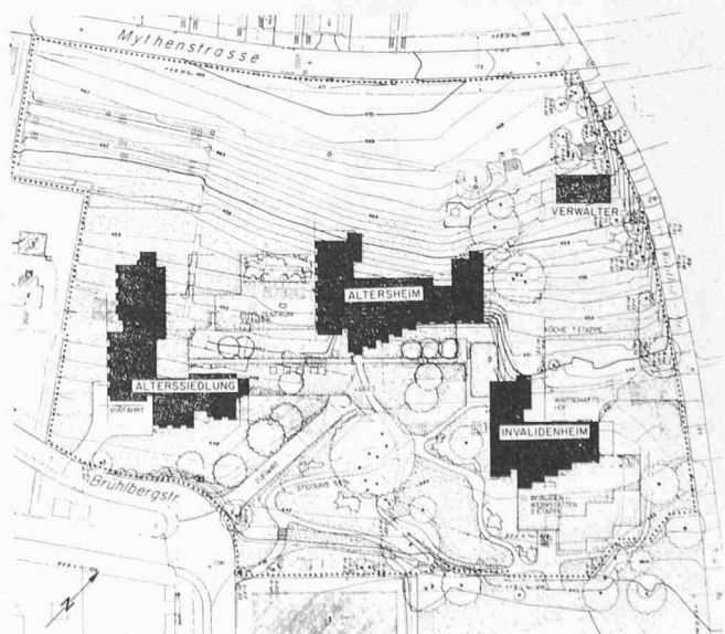
Lageplan 1:2500
