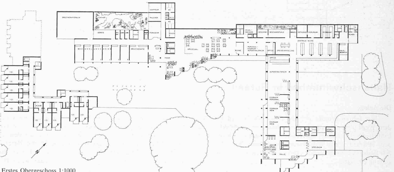
Erstes Obergeschoss 1:1000
