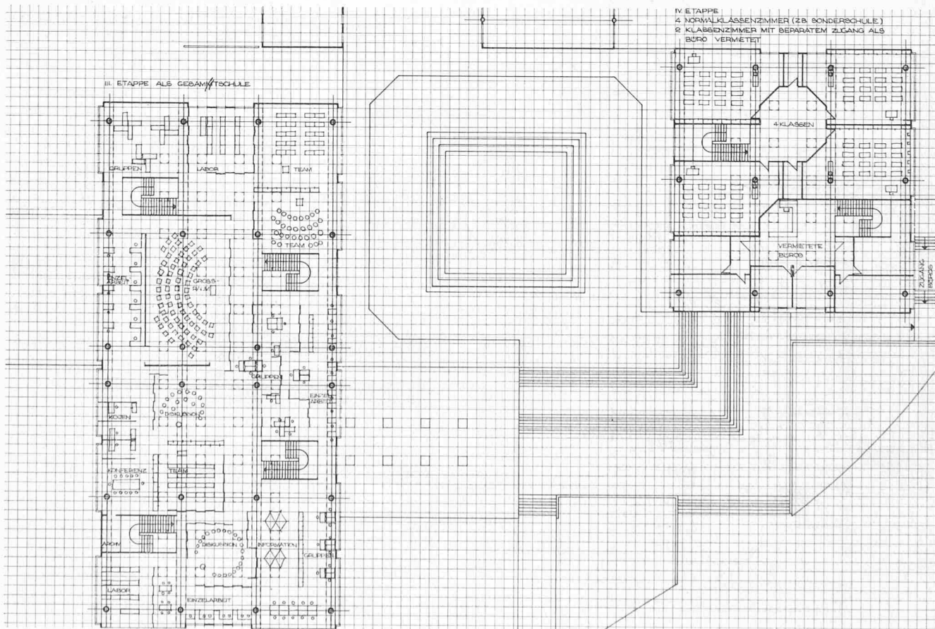
Nutzungsvarianten 1:600
