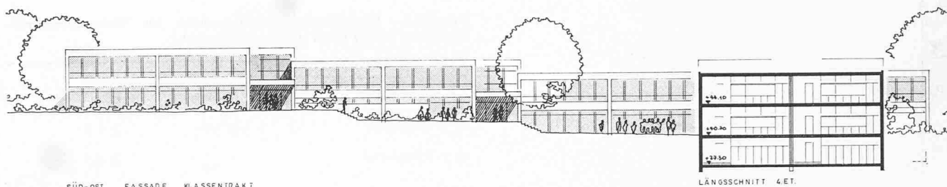
Südostfassade Klassentrakt und Längsschnitt 1:600
