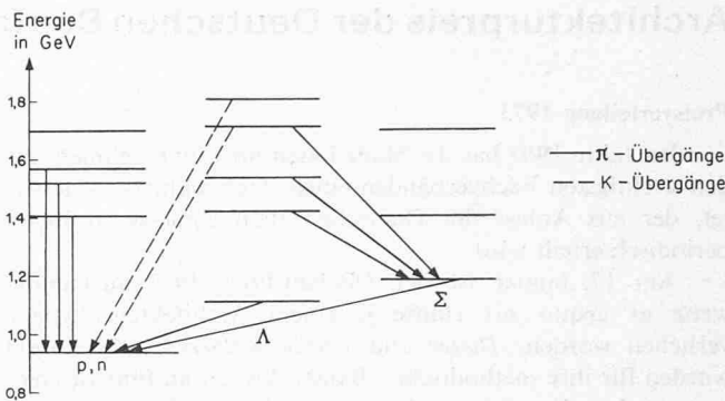
Bild 10. Baryonenspektrum
