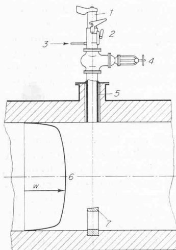
Heisswind-Temperaturmessungseinrichtung zur berührungslosen pyrometrischen Messung der Temperatur des Hochofen-Heisswindes
