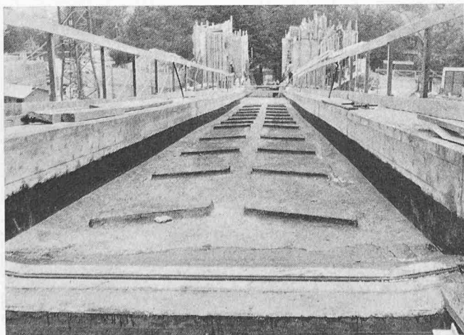
Bild 5. Innenansicht des Brückentroges im Bauzustand. Man erkennt die Nocken gegen das Wandern des Schotterkörpers und die Fahrbahnisolation mit Bitumenanstrich. Vorne der Fahrbahnübergang Widerlager 5 vor dem Einbau des Schutzbleches
