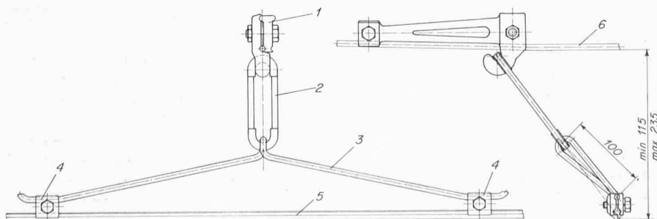
Bild 2. Elastische Aufhängung des Fahrdrabtes. 1 Gelenkbügel, 2 Isolierschlinge, 3 Stahlbügel, 4 Klemme, 5 Fahrdrabt, 6 Aufhangedraht quer zur Fahrtrichtung
