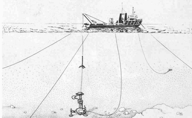
Bild 1. Zeichnung der Unterwasser-Bohreleinrichtung Maricor. Die Bohrkörner werden in einem Behälter (Bild 3) zum Schiff hochgezogen. Die Bohreinrichtung (Bild 2) wird vom Schiff aus ferngesteuert. Vier Verankerungskabel halten das Mutterschiff in Position
