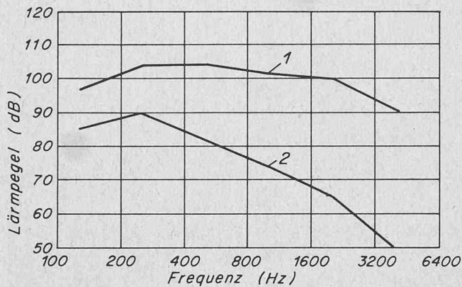
Dämpfungsspektrum des Schalldämpfers DIHF 200 über die Frequenz 1 Lärmpegel vor dem Schalldämpfer, Heizungsseite 2 Lärmpegel nach dem Schalldämpfer, Aussenseite
