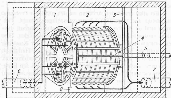
Bild 1. Durchflussschema einer Microstraineranlage (perspektivische Draufsicht). 1 Einlaufkammer, 2 Filterwasserkammer, 3 Ablaufwehr, 4 Spülwasserzulauf, 5 Spülwasserablauf, 6 Zulauf, 7 Ablauf, 8 Notüberfall
