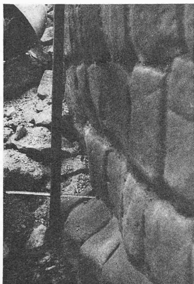
Bild 18. Schäden an der Wehrverkleidung der Fassung am Rio Pativilca nach der ersten Regenperiode. Die zwei unteren Blockreihen wurden gegen 20 cm abgeschliffen
