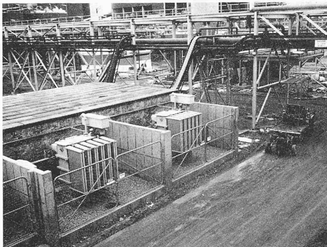
Bild 4. Transformerverteilstation mit Kabelverlegung auf Rohrbrücken
