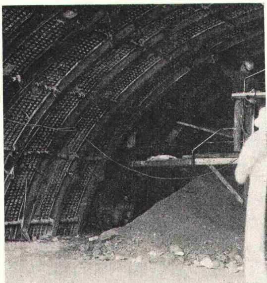
Tunnelauskleidung mit Schalungs- und Armierungsblechen Bernold®
