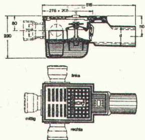
Kellerablauf «Junior» mit Rückstaudoppelschluss
