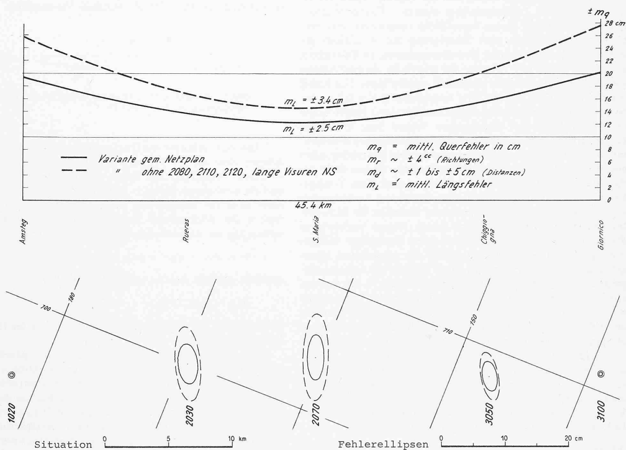
Bild 4. Einflusscharakteristik des Netzes auf den mittleren Querfehler unter beliebigem Durchschlagsort bei einer Absteckung von den Portalen aus (oben). Fehlerellipsen der Schachtanschlüsse bezüglich der Portalpunkte 1020, 3100 (unten)
