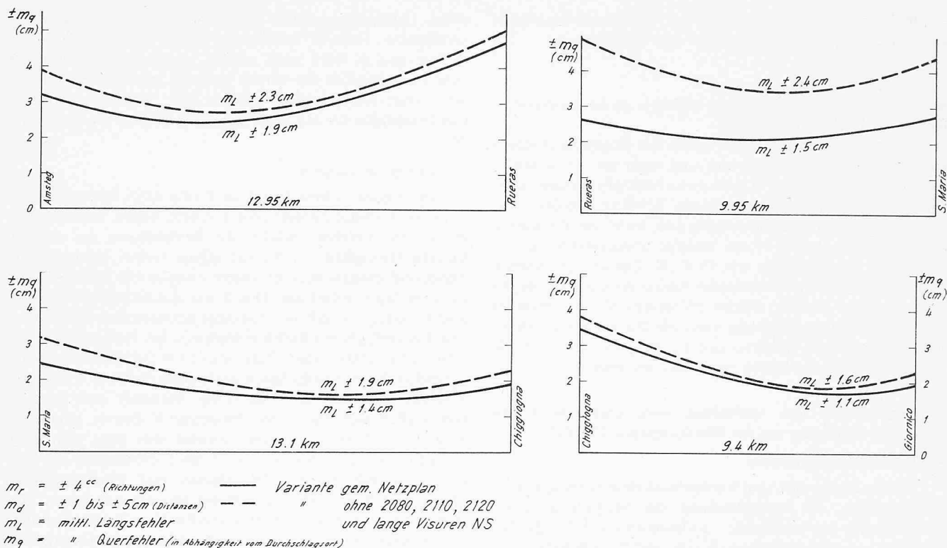
Bild 3. Einflusscharakteristik des Netzes auf den mittleren Durchschlagsfehler in Querrichtung für die Bauabschnitte bei beliebigem Durchschlagsort zwischen den Angriffsstellen
