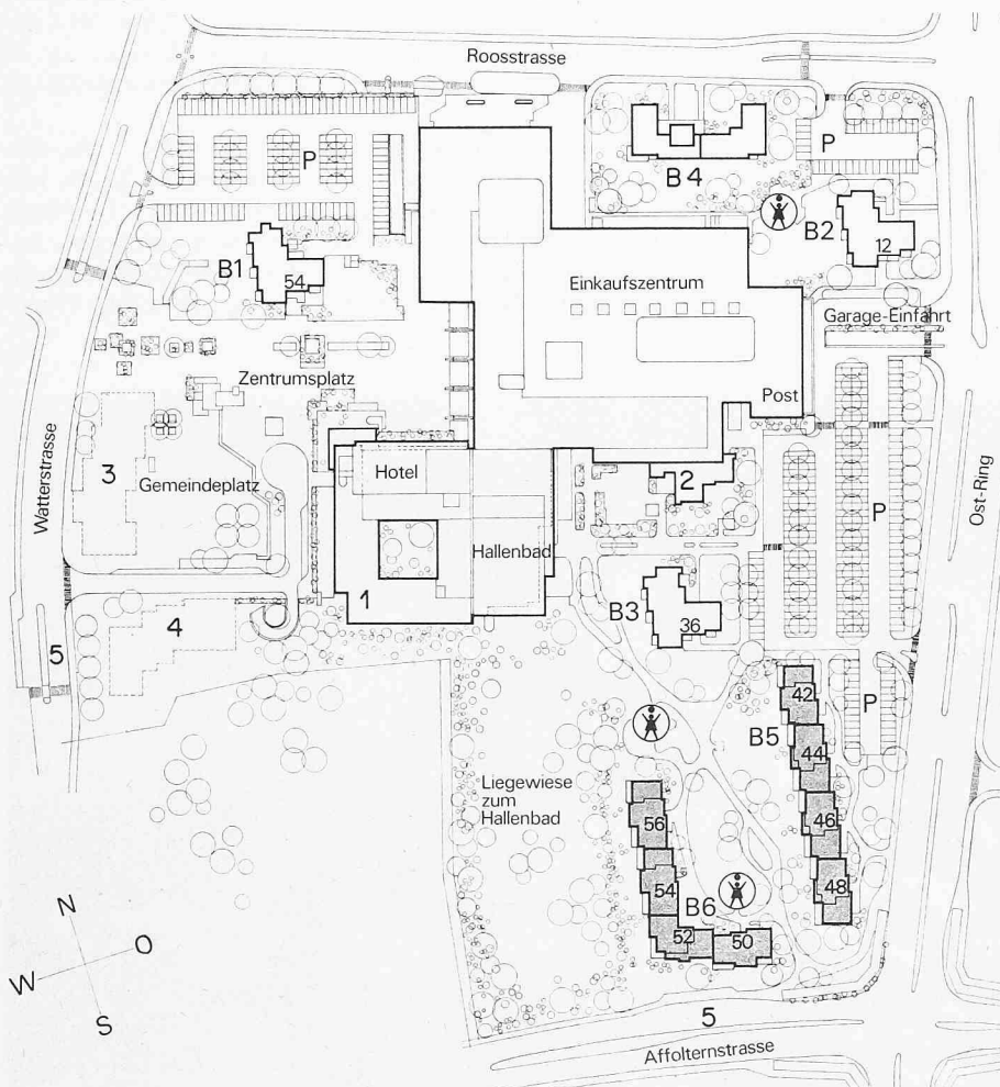
Gesamtplan 1:3000 der Zentrumsanlage Regensdorf B1, B2, B3 Wohnhochhäuser, B4 Personalhaus Mövenpick, B5, B6 Reihenhäuser (4. Bauetappe), Ost-Ring/Affolterstrasse. 1 Einkaufszentrum mit: EPA-Filiale, Migros-Supermarkt, LVZ-Center, BP-Auto-Center und 16 Spezialgeschäften und Bankfiliale SBG, 2 Post, 3 projektierter Kindergarten, 4 Hotel und Restaurant (Mövenpick Holiday Inn), 5 Hallenbad und Saal, 6 projektierter Gemeindeverwaltung, 7 projektierter Kirchgemeindehaus, 8 Bushaltestellen, 9 Einfahrt zur unterirdischen Autocinstallhalle
