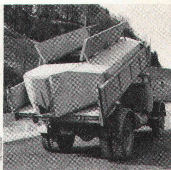
TIMPEX Warmhaltesilo für Belagsmisch- gut bei Handeinbau, Fassungs- vermögen ca 7 t
