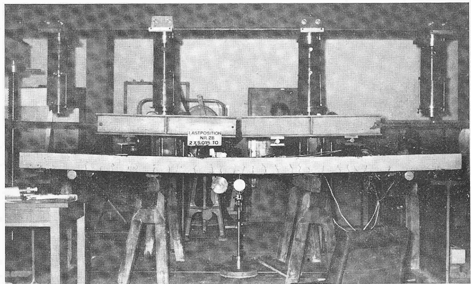
Bild 10. Versuchsplatte mit geklebter Biegearmierung unter Last
