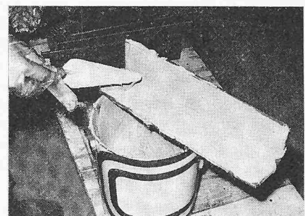
Bild 34. Auftragen der Klebmasse auf die Stahlteile
