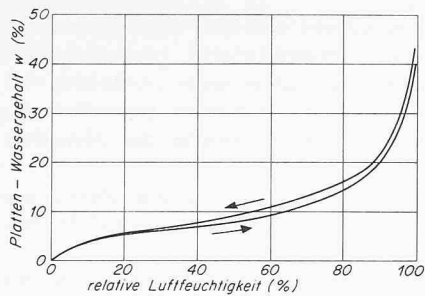
Bild 2. Mittlere Wasserdampf-Sorptionsisothermen für t = 20^\circ\text{C}
