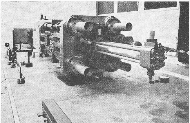
Bild 2. Testaufbau im Holographielabor für Objekte bis 4000 kg bei Brown Boveri (Photos Brown Boveri)
