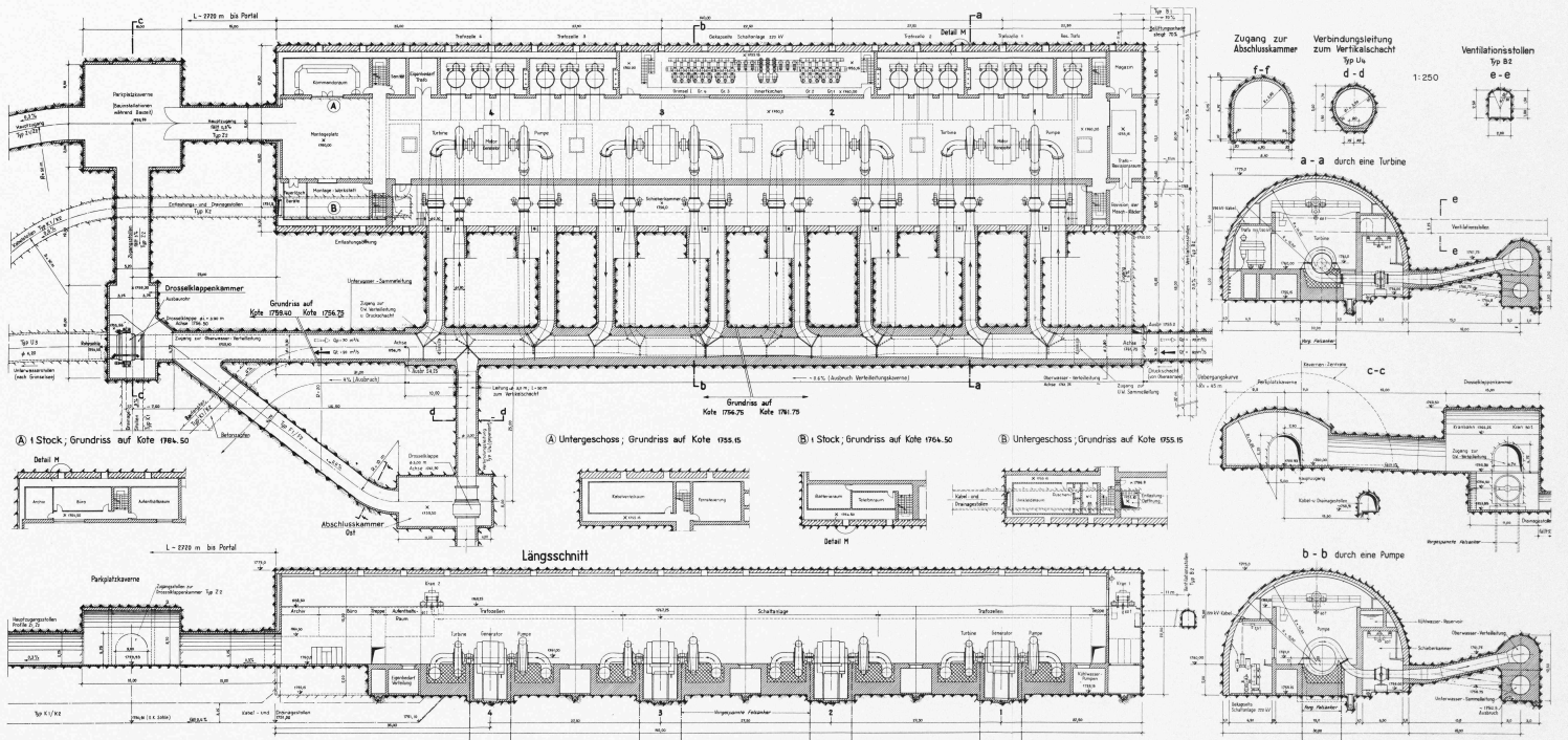
Zentrale Grindel II Ort der Kraftwerk Oberhall AG, Grundriss und Schnitte 1:500
