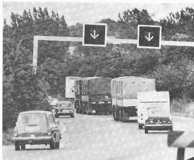
Lichtzeichenanlage auf einer Autobahn am Dreieck Köln-Heumar
