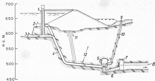
Bild 3. Längsschnitt der Kraftanlage G.M. Shrun. 1 Einlaufkontrolle, 2 und 3 Einlauf, 4 Druckrohre, 5 Maschinenhaus, 6 Auslass, 7 und 8 Ausgleichskammer und Ablasskanal, 9 Umspannstation, 10 Kabelschacht, 11 Abschrägung, 12 Entwässerungstunnel
