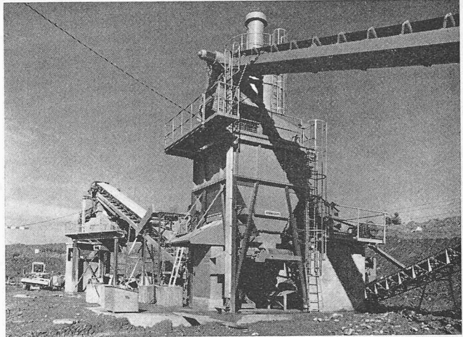
Bild 4. Die Stabilisierungszentrale des Bauloses «Umfahrung Rütli» weist eine Abgabeleistung von 80 bis 100 m 3 /h verdichtetem Material auf. Mit einem zweiten Mischer ausgerüstet, erreicht sie mindestens 150 m 3 /h (Werkbilder AMMANN, Langenthal)
