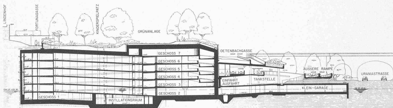
Schnitt 1:800
