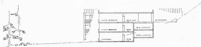
Schultrakt, Querschnitt 1:800
