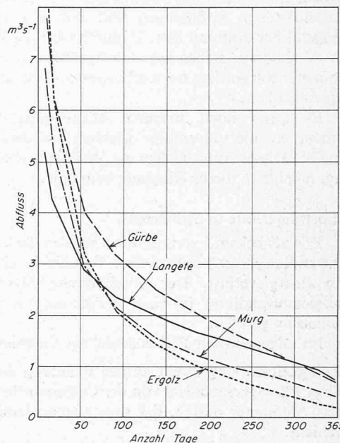
Bild 4. Vergleiche von Abflussdauercurven
