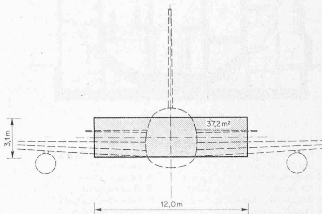
Bild 10. Flugzeugabsturz. Aufprallfläche
