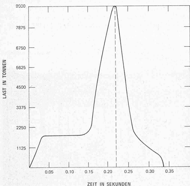
Bild 9. Last-Zeit-Funktion für den Lastfall Flugzeugabsturz gemäss Riera [2]
