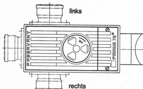
Primus 70 3fach gesicherter Kellerablauf gegen Rückstau
