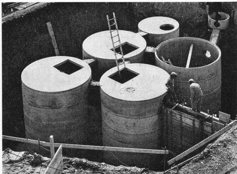
Einbau einer biologischen Kläranlage im Kanton Schaffhausen (320 EWG)
