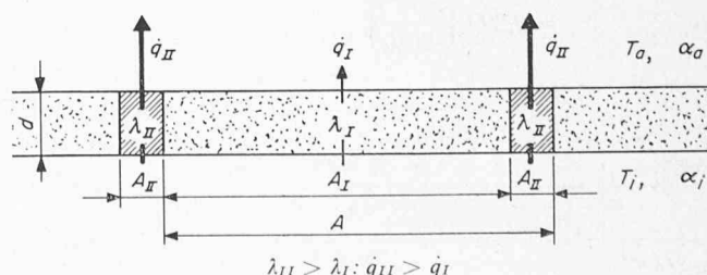
Bild 1. Wärmebrücke
