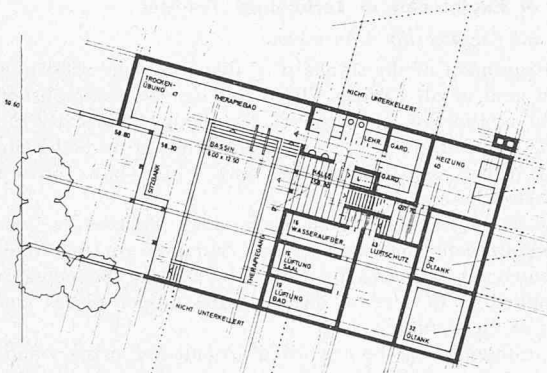
Grundriss Untergeschoss 1:700
