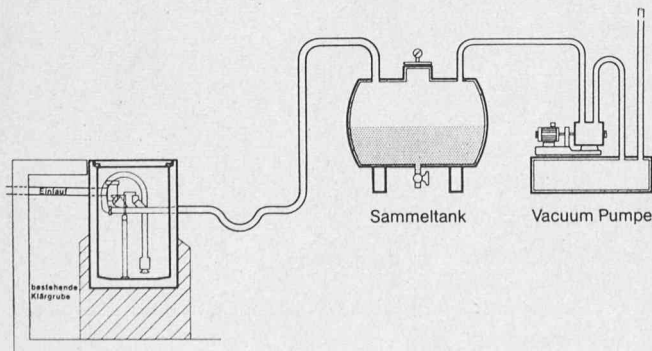
Vacuflow-Absauganlage
