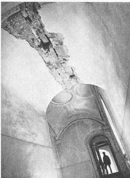
Bild 6. Gewölberisse über den Seitengalerien mit Durchblick zur Turmtreppe (vgl. Querschnitt Bild 4)
