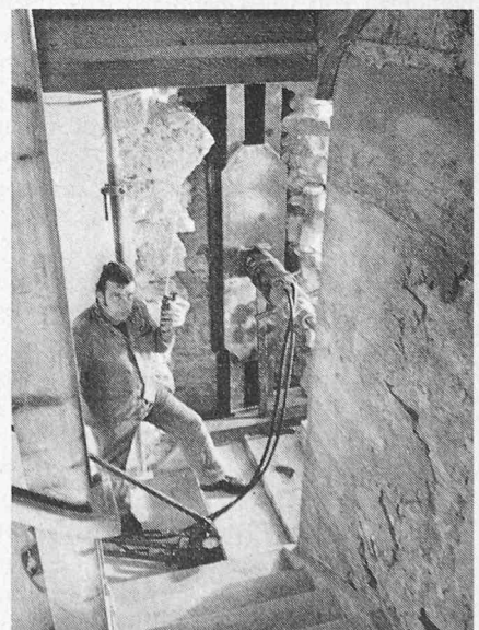
Bild 8. Auswechslung des Kabels A bei der Turmtreppe. Funkgerät zum Koordinieren der Pressen an beiden Enden des U-förmigen Kabels
