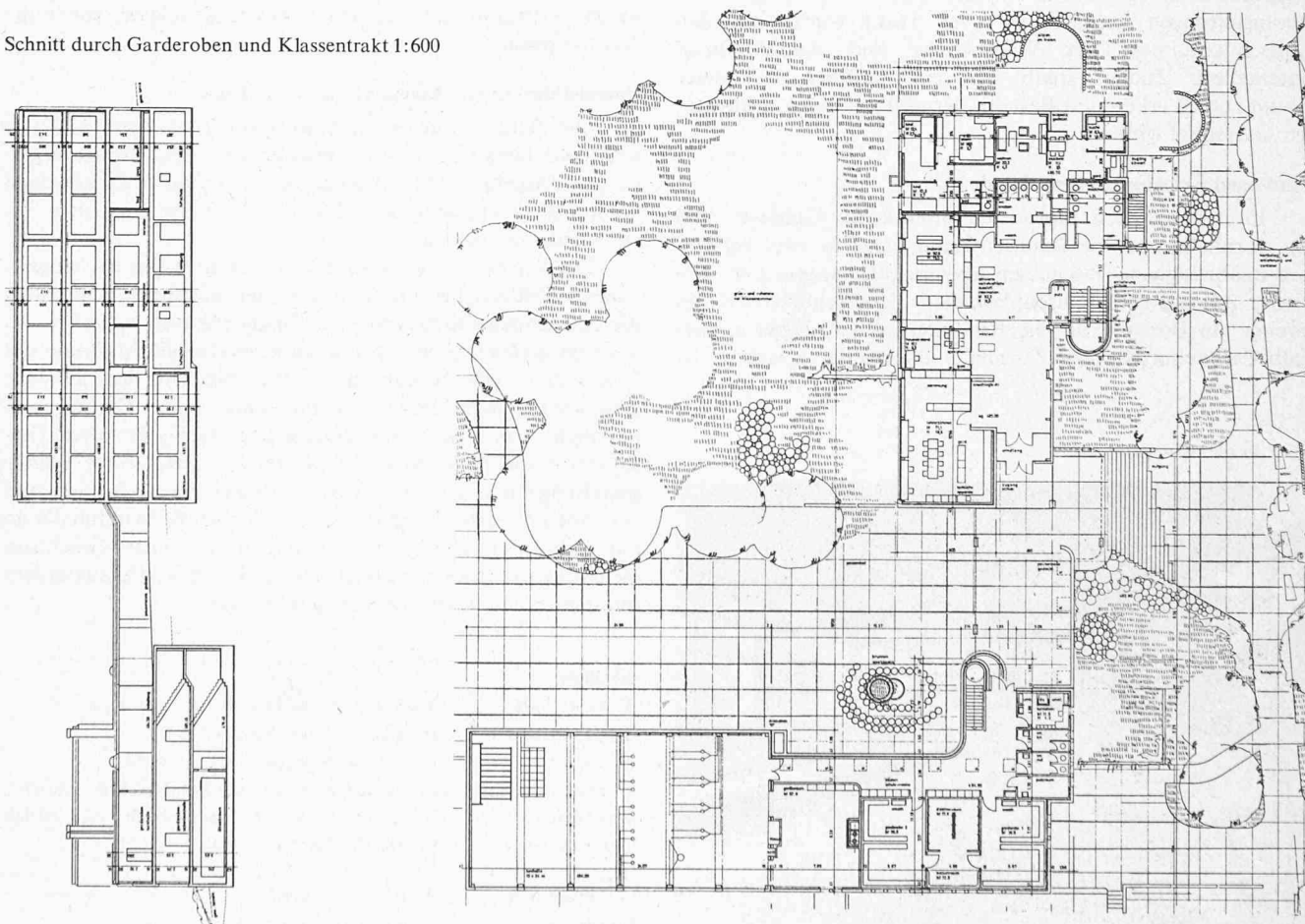
Grundriss Erdgeschoss 1:600
