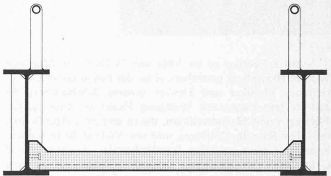
Querschnitt der Fussgängerbrücke über die Murg
