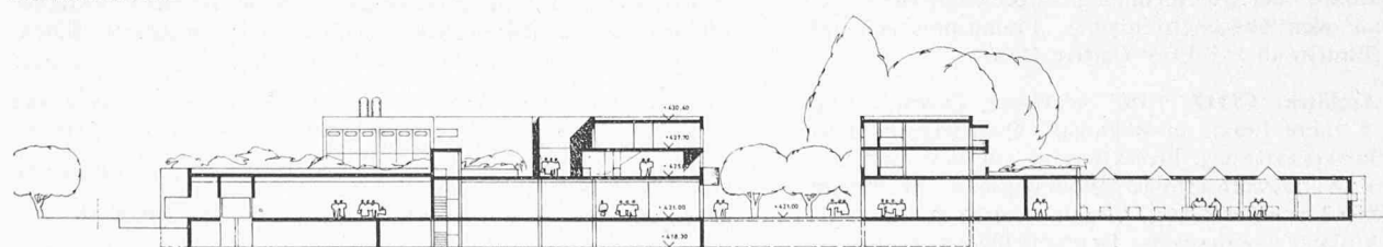
Schnitt 1:800
