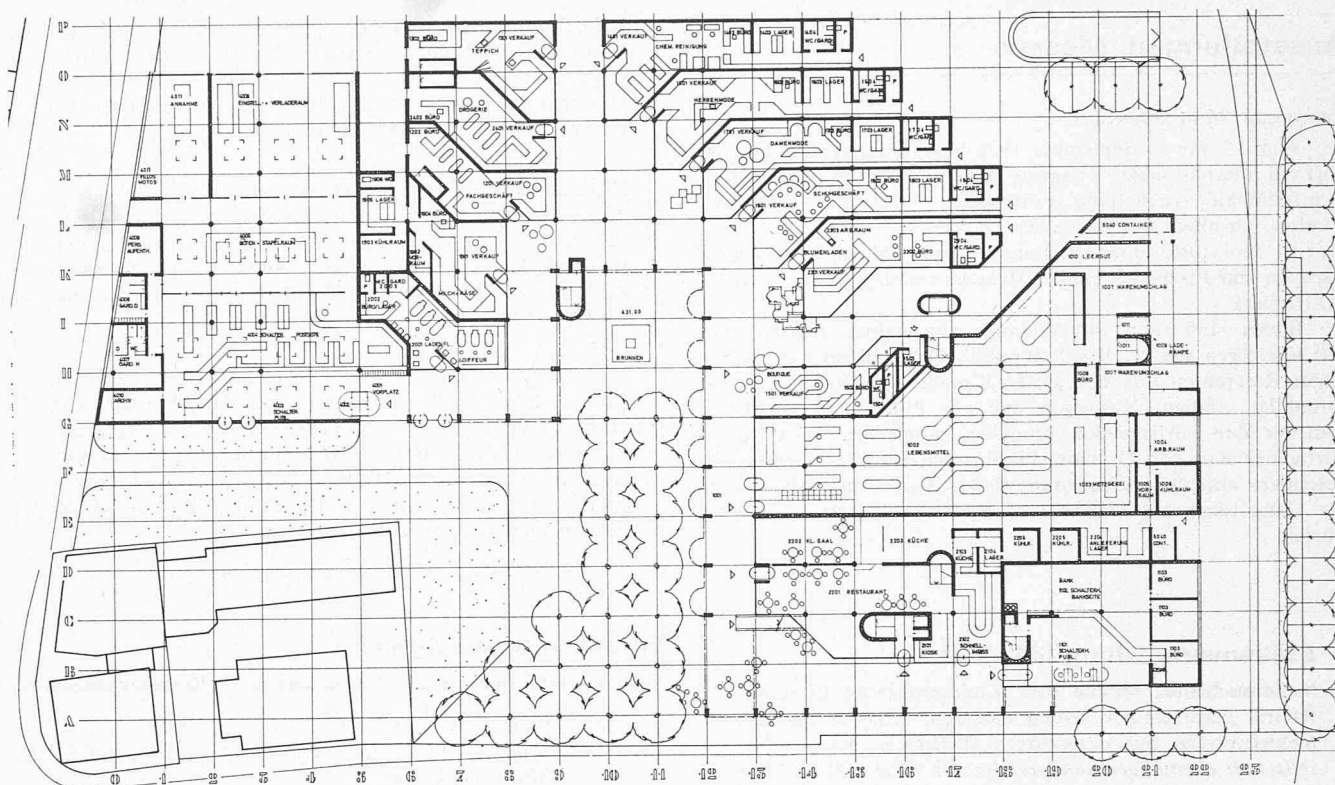
Erdgeschoss 1:800
