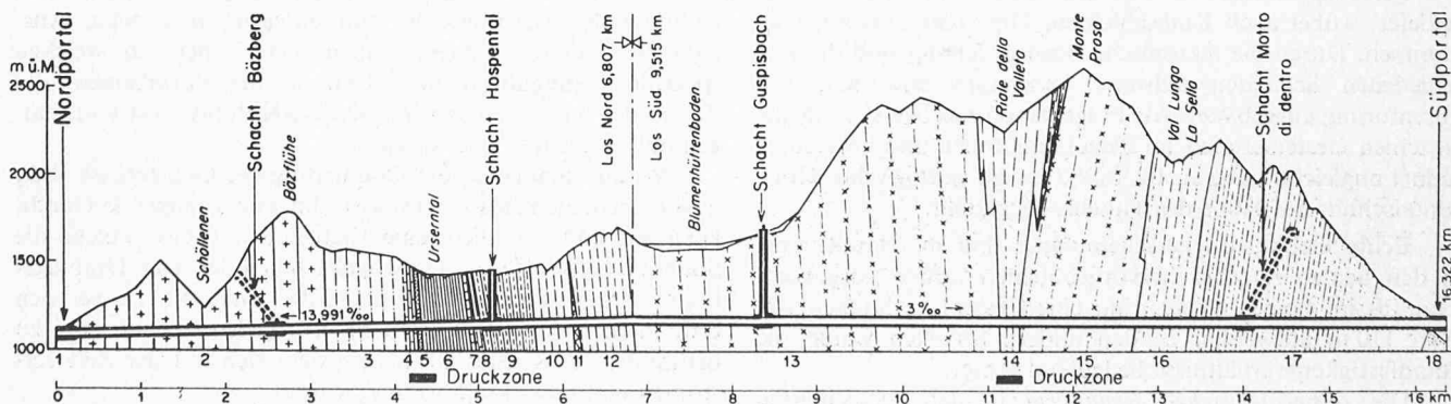
Bild 1. Geologisches Längenprofil
