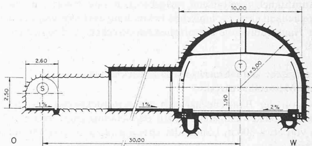
Bild 2. Querprofil Tunnel (T) und Sicherheitsstollen (S)
