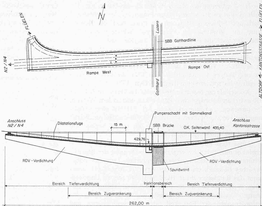
Bild 1. Übersichtsplan des Bauwerkes mit den Zubringern
