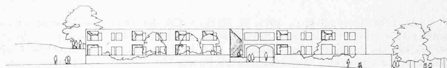
Südostansicht 1:800. Alterswohnungen
