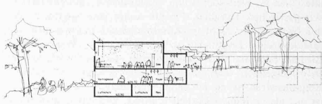
Schnitt durch Sakralraum 1:800
