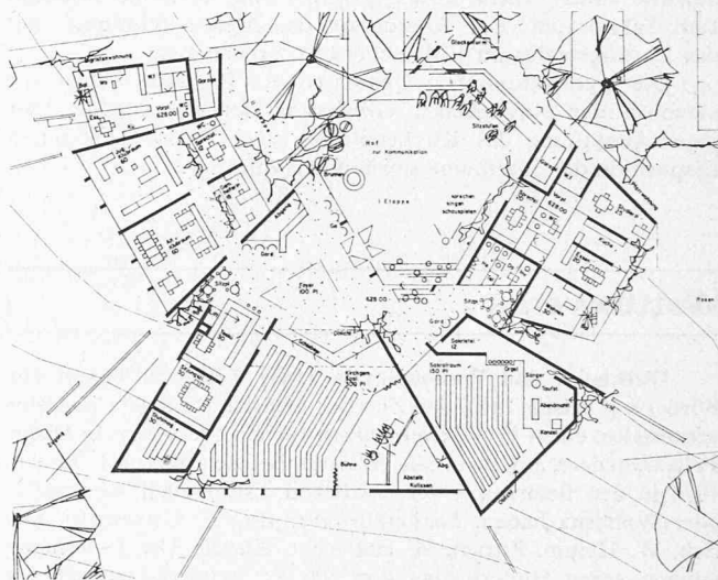
Grundriss Eingangsgeschoss 1:800
