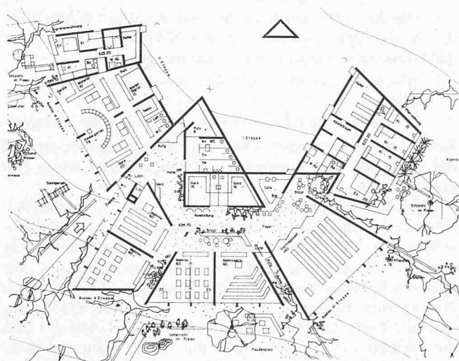
Grundriss Erdgeschoss 1:800
