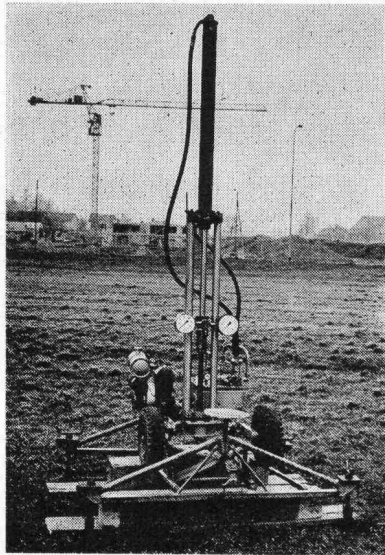
Holländische Drucksonde
